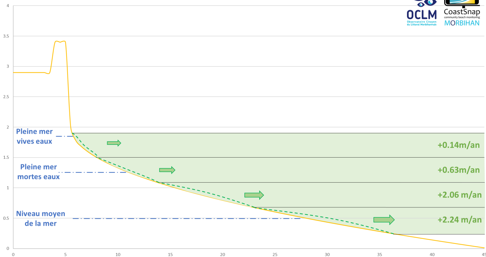
Tendances d'évolution du profil de la plage de la falaise (ARZ)
